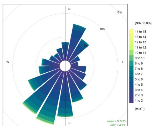
Rose des vents à MétéoFrance Saint-Hilaire du 01/01/2023 à 00h00 (TU) au 01/01/2024 à 00h00 (TU) (données horaires)
