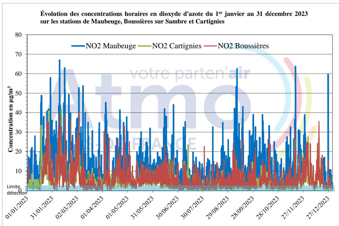
Figure 9 : Graphe des concentrations horaires en NO 2
